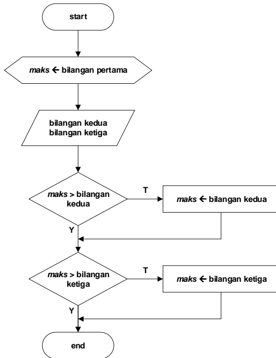
Gambar. Contoh Penulisan dengan Flowchart
